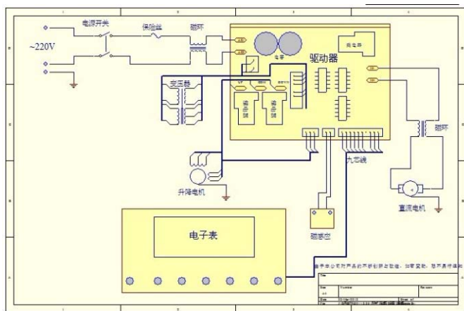
电路图
